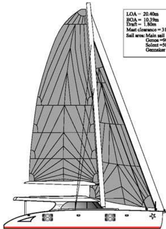
Voilure
